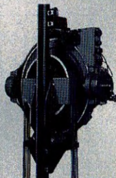
Сучасний привод ліфта фірми Kone з малогабаритною безредукторною лебідкою EcoDisc. Привід від синхронного двигуна зі збудженням на постійних магнітах.
