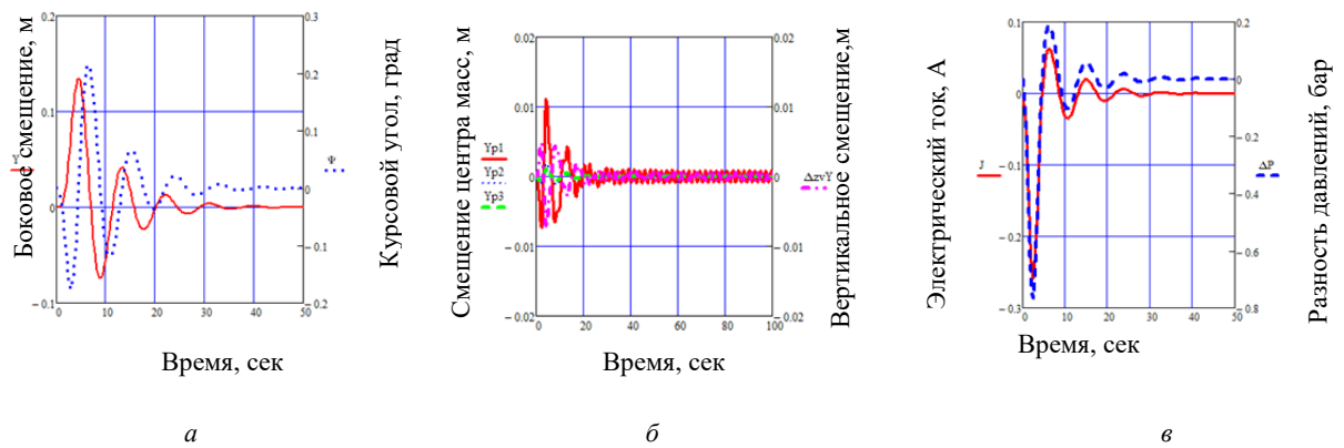
Рис.14. Быстрое восстановление курса при K_\psi = 1000\text{В}, K_\omega = 2000\text{Вс}, K_y = 50\text{Вм}^{-1} а – изменение курсовых параметров; б – колебания парциальных осцилляторов; в – колебания параметров регулятора
