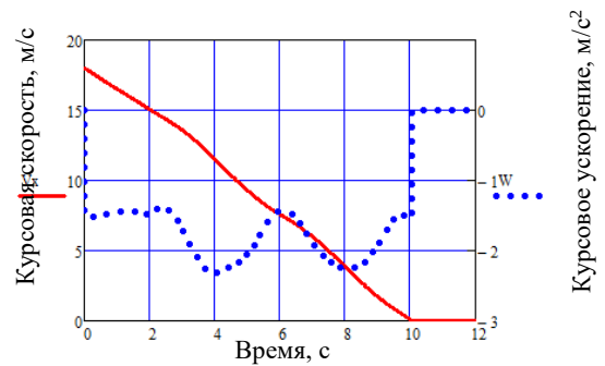
Рис. 2. Параметры торможения топливозаправщика КраЗ-63221 с цистерной АПЦ-20
