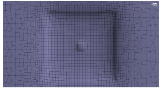
Рис. 1. Вигляд скінчено-елементної моделі зверху: півпростір під дією тиску штампу \frac{a}{b} = 0.1
