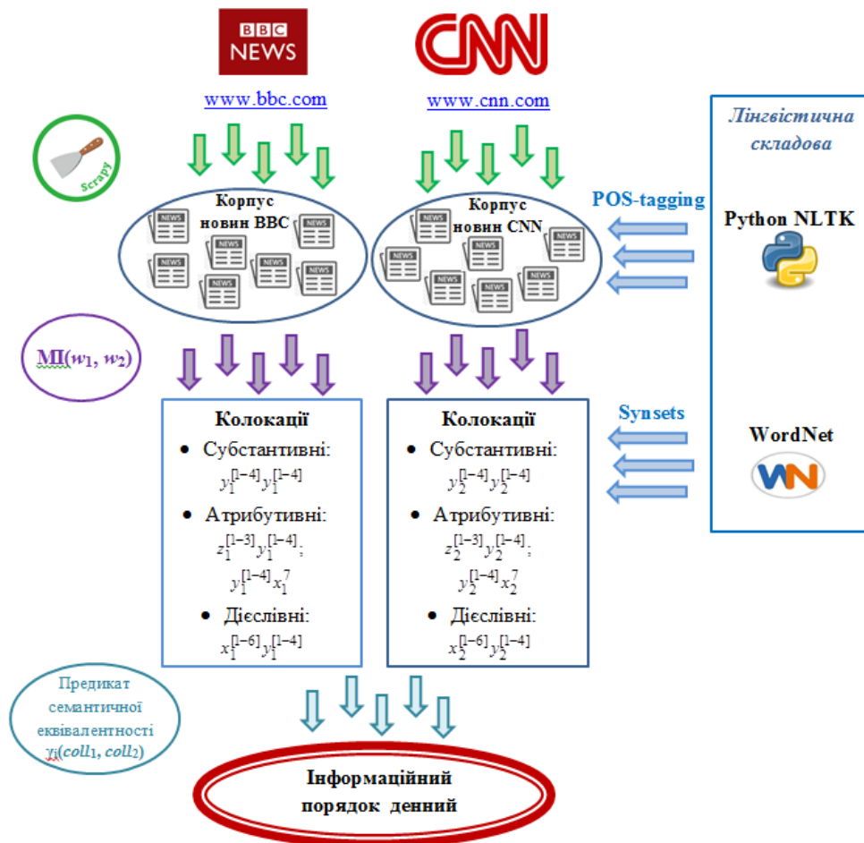
Рис. 1. Етапи інформаційної технології визначення інформаційного порядку денного в потоках новинних даних
