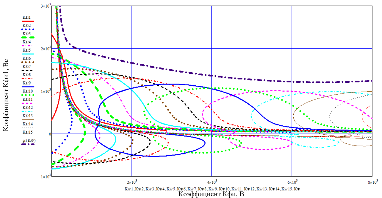
Рис.15. Актуальный участок нижней границы области курсовой устойчивости при частотах 0–0.4 Гц и значении K_y = 50\text{Вм}^{-1} . Пре среднем уровне жидкости h_* = 0.7\text{м} скорость автомобиля снижена до 12м/с, а штрихпунктирная линия является границей области устойчивости для V_* = 18\text{м/с}
