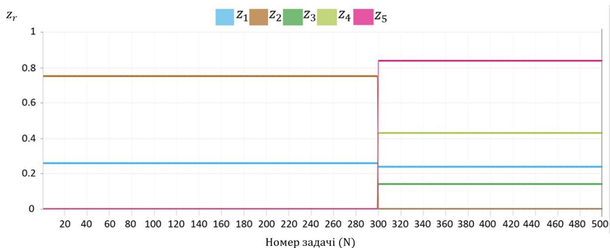
Рис. 4. Результати експерименту типу 2 для задачі на мінімум
