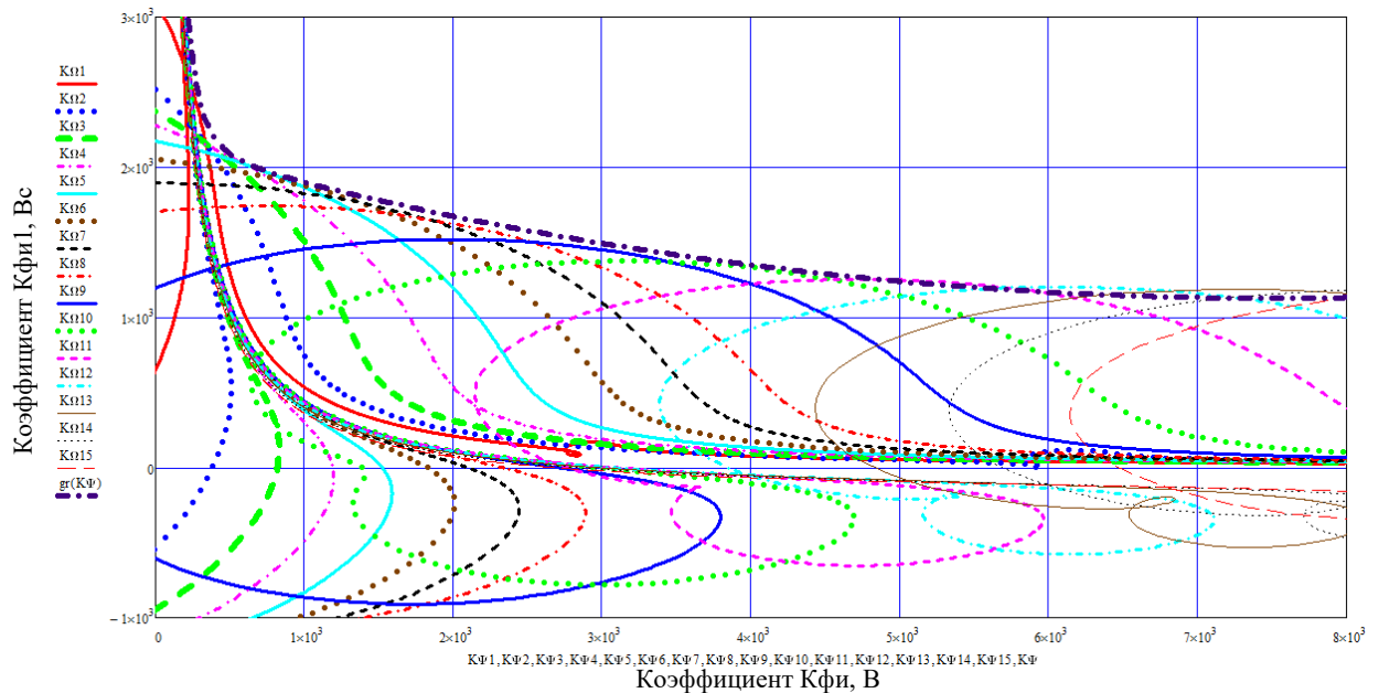
Рис. 10. Актуальный участок нижней границы области курсовой устойчивости при частотах 0–0.4 Гц и значении коэффициента K_y = 50 \text{ Вм}^{-1} . Штрихпунктирная линия огибает все траектории сверху и создает указанную границу
