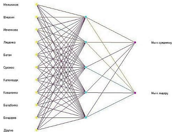
Рис. 3. Граф нейронной сети MLP-11-5-2
