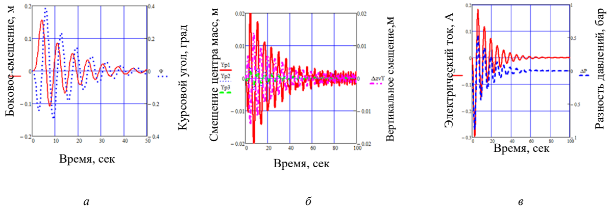
Рис. 13. Медленные переходные процессы при K_\psi = 1000\text{В}, K_\omega = 1000\text{Вс}, K_y = 50\text{Вм}^{-1} : а – изменение курсовых параметров; б – колебания парциальных осцилляторов; в – колебания параметров регулятора
