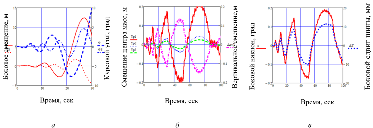
Рис. 12. Неустойчивый процесс движения при K_\psi = 1000\text{В} , K_\omega = 300\text{Вс} , K_y = 50\text{Вм}^{-1} : а – изменение курсовых параметров (буква S соответствует «отвердевшему» грузу); б – колебания парциальных осцилляторов; в – боковые колебания корпуса автомобиля
