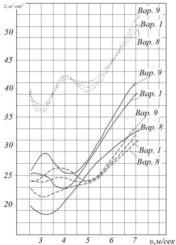
Рис. 4 – Значення середньоквадратичних прискорень точок остова для різних жорсткостей передньої підвіски під час руху трактора по природним нерівностям 2k_1 = 34 \text{ кН} \cdot \text{с/м} :
