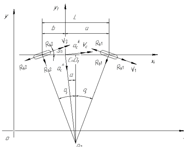
Рис. 2. Схема сил, які діють на автомобіль з усіма керуючими колесами при повороті їх в різні сторони
