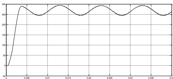
Рис. 10 - Напруга на накопичувальному конденсаторі силового активного фільтра
