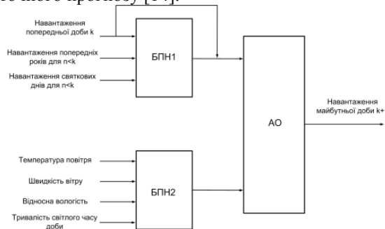
Рисунок 2 – Блок-схема багатошарової штучної нейронної мережі ANNSTLF
