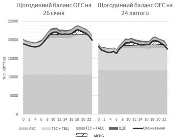
Рисунок 6 – Участь електростанцій ОЕС у покритті графіку навантаження
