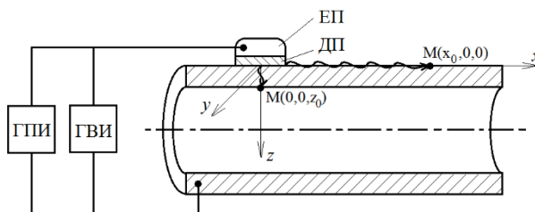
Рис. 1 – Распространение продольной волны вдоль оси z и поверхностной волны вдоль оси x : M(x_0, 0, 0) – точка наблюдения с координатами (x_0, 0, 0) ; M(0, 0, z_0) – точка наблюдения с координатами (0, 0, z_0) .
