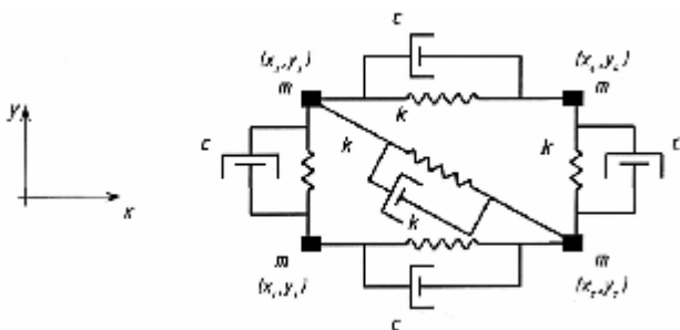
Рис. 3. Площа прямокутна ферма m = 100,0 \text{ кг} ; k = 36,0 \text{ Н/м} ; c = 45,0 \text{ Н} \cdot \text{с/м} .
