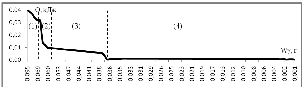
Рисунок 2 – Енергетична крива процесу сушки, характерної для листвяних порід, на прикладі берези
