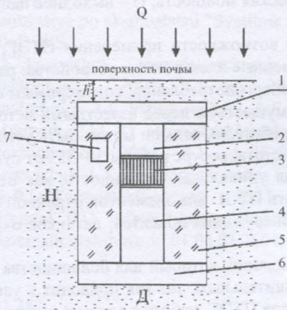
Рисунок 1 – Схематическое изображение ПТЭГ
