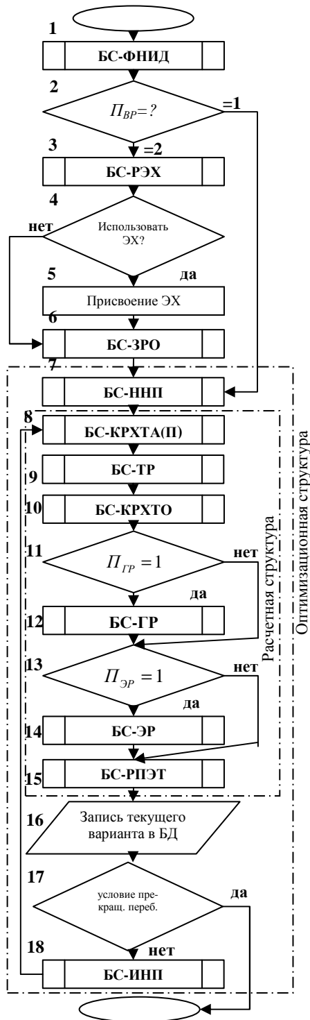
Рисунок 1 – Структура синтезатора алгоритмов оптимизации и оптимальной замены кожухотрубчатых и пластинчатых теплообменников (ОПКТО–2014)
