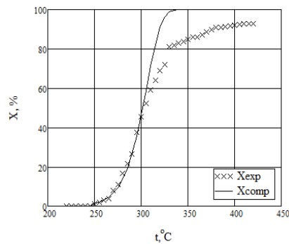
Рисунок 7 - Расчетная X_{comp} и экспериментальная X_{exp} зависимости степени конверсии углеводородов от температуры
