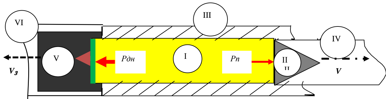
Рисунок 3 – Рабочий процесс в двигателе автоматики
