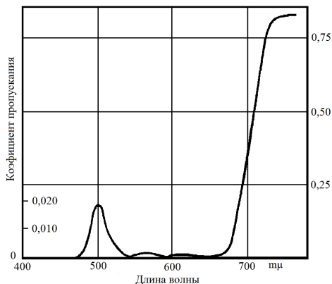
Рисунок 4 – Спектральная кривая пропускания цветоконтрастных светофильтров для зелени На рисунке 4 масштаб коэффициента пропускания для волн короче 680 \text{ м}\mu увеличен в 10 раз. Такие
