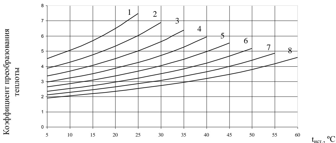
Рисунок 1 – Зависимость коэффициента преобразования энергии μ от температуры низкопотенциального источника теплоты t ист. и температуры теплоносителя t тн. нагретого в тепловом насосе
