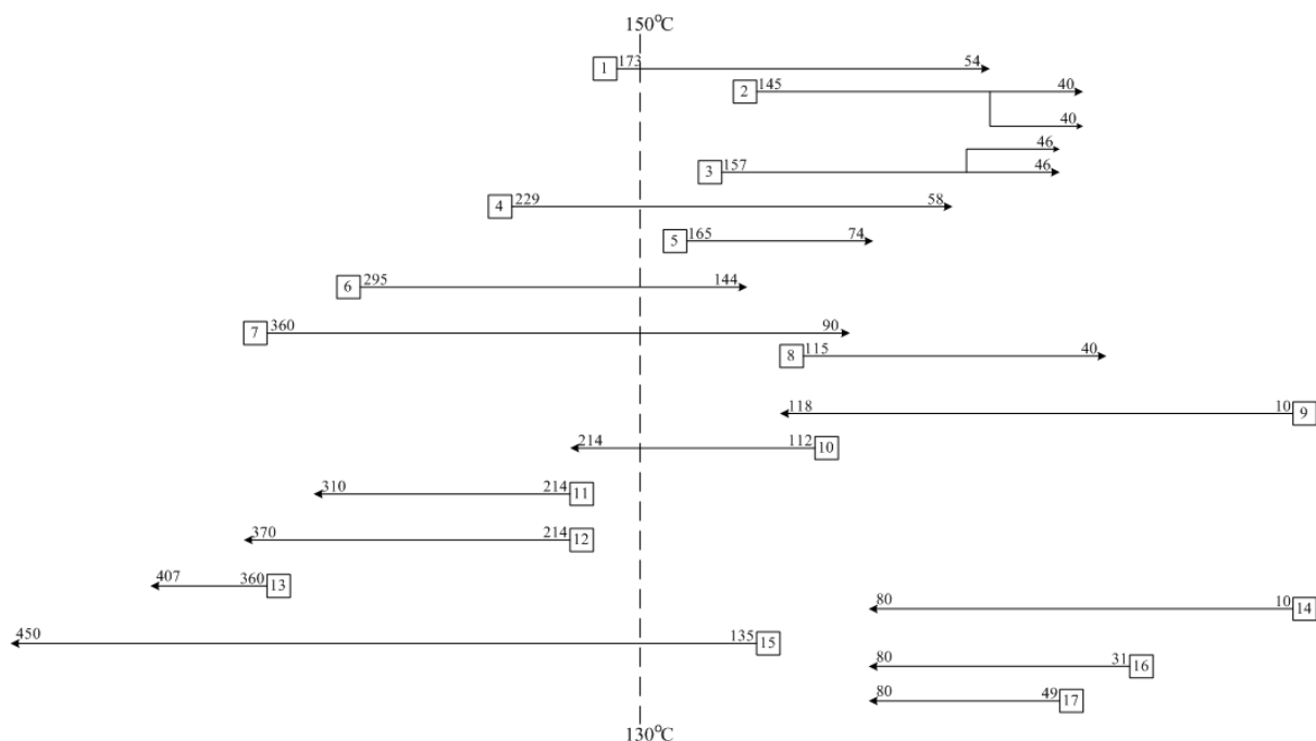
Рисунок 3 – Популяция технологических потоков на установке АВТ А12/2 в режиме работы без вакуумного блока
