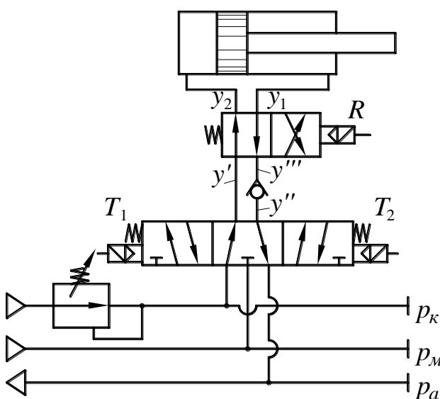
Рисунок 6 – Энергосберегающая структура ПА (схема № 2)
