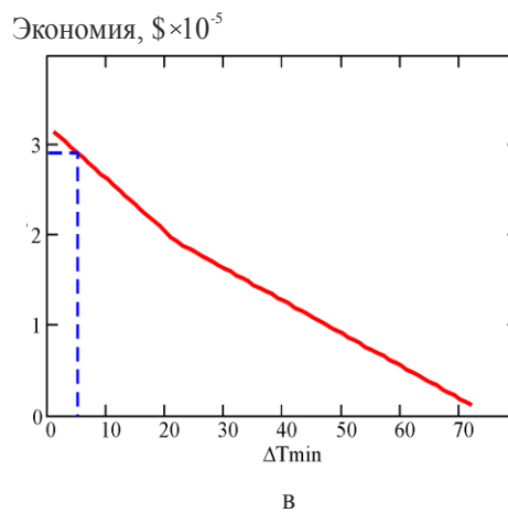
Рисунок 5 – Диаграмма соответствия между возможными целевыми функциями используемых для создания оптимизированных проектов реконструкции процесса концентрирования в производстве фосфорной кислоты экстракционным методом а – зависимость срока окупаемости от капитальных вложений; б – зависимость величины прибыли от капитальных вложений; в – зависимость величины прибыли от \Delta T_{min}
