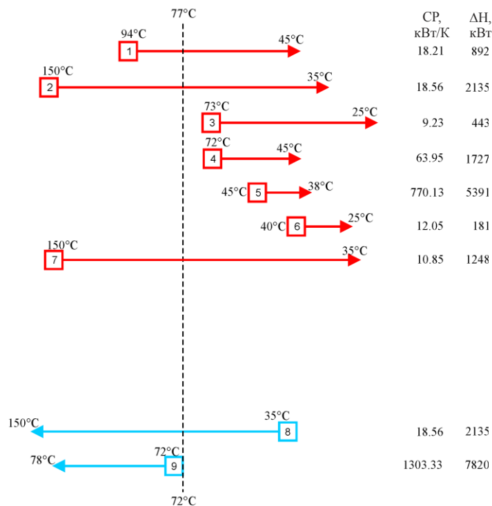
Рисунок 6 – Локализация пинча на популяции технологических потоков для технологического процесса, изображенного на рис. 1
