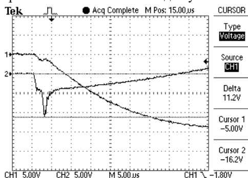
Рис. 1. Поеднані осцилограми струму i_c(t) (крива каналу 1) і напруги u_c(t) (крива каналу 2) в сильнотривому розрядному колі потужного високовольтного ГІС при ЕВ в атмосферному повітрі тонкого мідного провідника ( l_0 \approx 110 мм; r_0 \approx 0,1 мм; t_{ex} \approx 3,2 мкс [30]) (масштаб за вертикаллю для струму – 50 кА/поділку; масштаб за вертикаллю для напруги – 12,6 кВ/поділку; масштаб за горизонталлю – 5 мкс/поділку)
