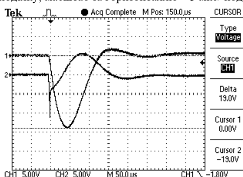
Рис. 2. Ті ж, що й на рис. 1 суміщені осцилограми розрядного струму i_c(t) (крива каналу 1; I_{mc} \approx 190 кА; \delta_c \approx 14,39 \cdot 10^3 с -1 ; \omega_c \approx 26,18 \cdot 10^3 с -1 ; T_c \approx 2\pi/\omega_c \approx 240 мкс [30]) і напруги u_c(t) (крива каналу 2) в сильнотривому розрядному колі потужного високовольтного ГІС при ЕВ в атмосферному повітрі тонкого мідного провідника ( l_0 \approx 110 мм; r_0 \approx 0,1 мм; t_{ex} \approx 3,2 мкс) тільки при масштабі за горизонталлю – 50 мкс/поділку
