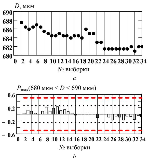
Рис. 5. Результаты контроля диаметра (а) эмальпровода в непрерывном технологическом цикле и контрольная карта максимальной вероятности выхода диаметра за границы нормативного диапазона (b)
