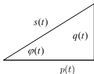
Рис. 2. Треугольник мгновенных мощностей
