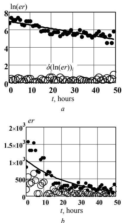
Рис. 1. Разделение массива данных о количестве дефектов на катушке (черные точки) на – детерминированную функцию f(t_i) (тренд: сплошная линия экспоненциальной функции) и случайную величину \delta_i (пустые точки) с помощью различных математических процедур разделения
