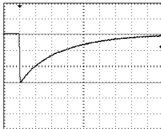
Рис. 6. Осциллограмма длительной С- компоненты тока искусственной молнии с нормированными АВП в сильноточной цепи генератора ГИТ-С при разряде его мощного ЕНЭ на воздушную ДЭС с электрически взрывающейся тонкой медной проволоочкой ( r_e = 0,1 мм; l_e = 37 мм) и листовым ИО из алюминиевого сплава марки АМг2М толщиной 2 мм ( U_{cc} \approx 4,2 кВ; W_C \approx 400 кДж; I_{mdc} \approx 0,869 кА; t_{mdc} \approx 9 мс; \tau_{pdc} \approx 1000 мс; q_{dc} \approx 192 Кл; масштаб по вертикали – 282 А/клетка; масштаб по горизонтали – 100 мс/клетка)
