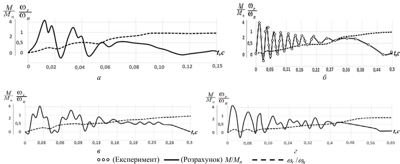
Рис. 4. Розрахункові та експериментальні осцилограми пуску АД при зміні статичного моменту для схеми S_{13}Z_{0}r_{11} : а – M_s = 0 , б – M_s = M_n ; та для схеми S_{13}Z_{0}r_{32} : в – M_s = 0 , г – M_s = M_n
