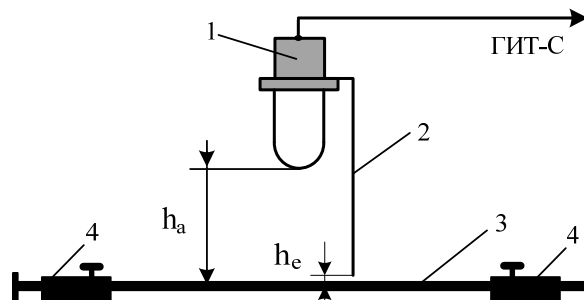
Рис. 4. Общий вид воздушной ДЭС в силовоточной разрядной цепи генератора ГИТ-С (1 – верхний массивный цилиндрический стальной электрод; 2 – круглая тонкая медная ЭВП; 3 – нижний массивный плоский электрод, являющийся ИО металлической обшивки технического объекта; 4 – массивные прямоугольные алюминиевые электроды, предназначенные для жесткого двухстороннего закрепления в их пазах плоского ИО; h_a – длина воздушного промежутка в ДЭС; h_e – длина воздушного промежутка между нижним краем медной ЭВП и наружной плоской поверхностью ИО)
