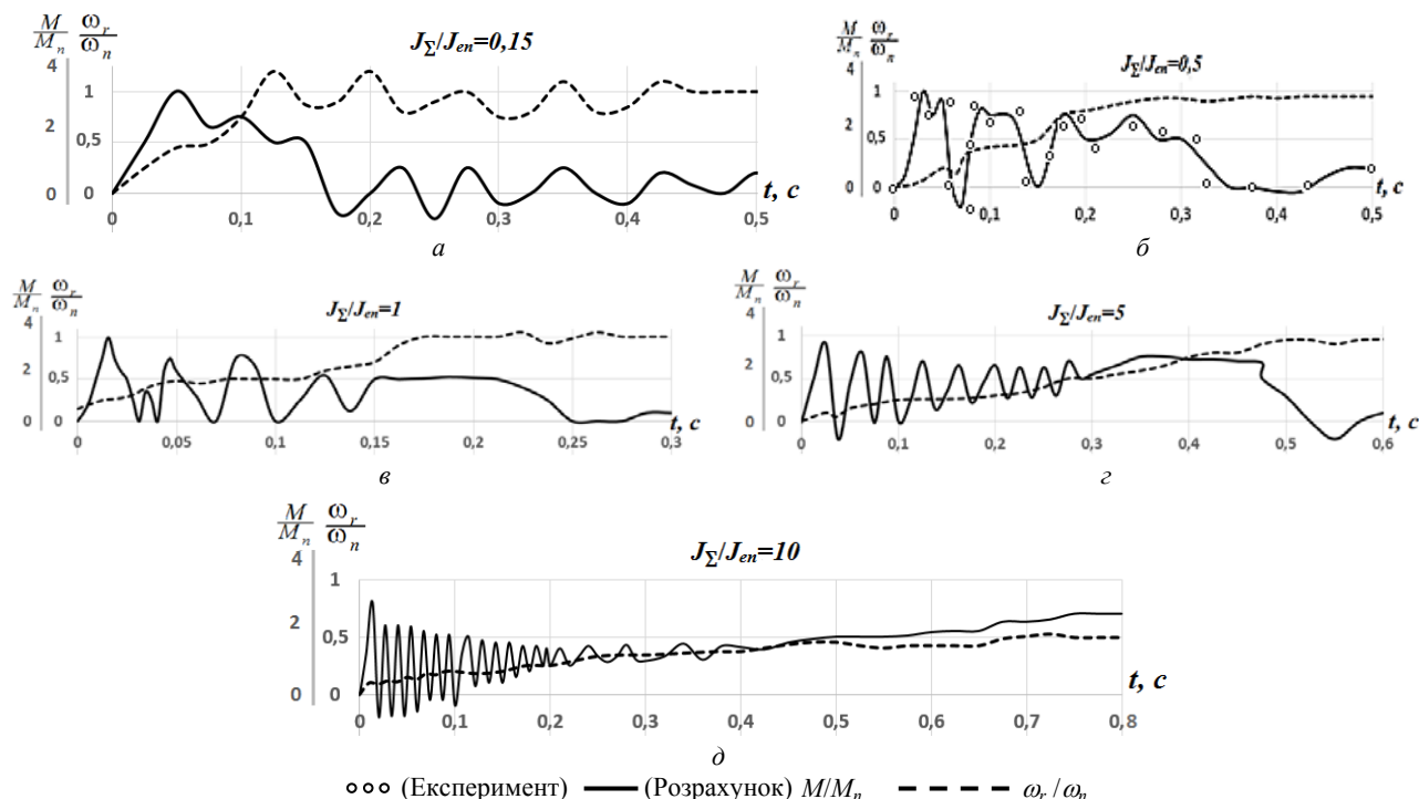
Рис. 3. Осцилограми пуску електроприводу з різними значеннями махових мас
