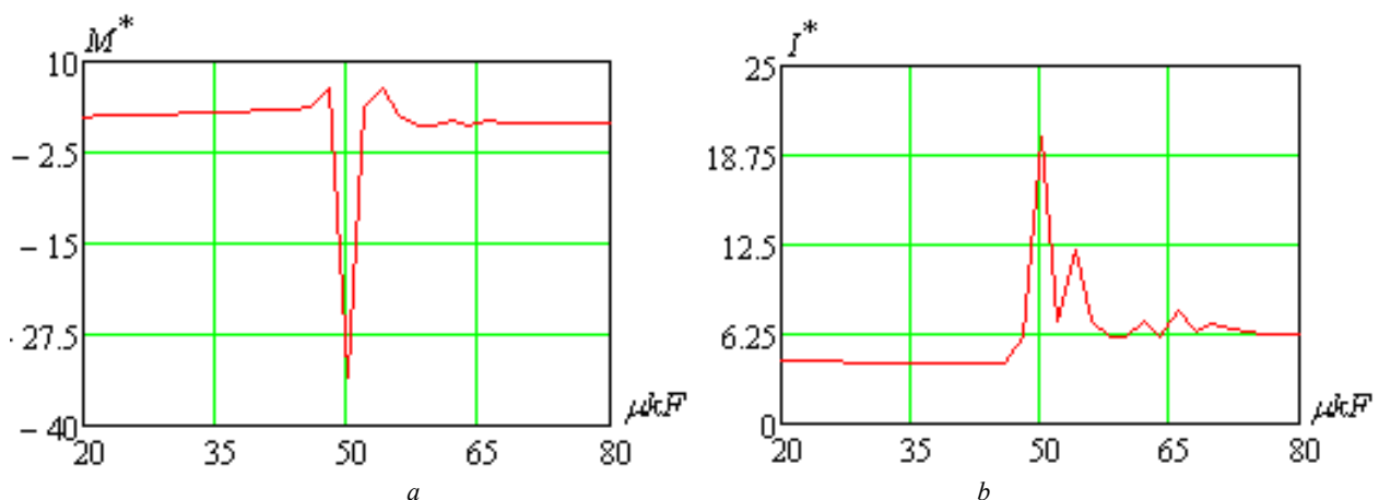
Рис. 1. Залежності рушійного ( s=1 ) електромагнітного моменту (а) та діючого значення струму якоря (б) від величини ємності конденсатора в обмотці збудження двигуна: а) C = 50 мкФ, б) C = 45 мкФ
