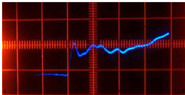
Рис. 8. Осциллограмма фронтальной части импульса напряжения на нагрузке ГИНПО в виде трех рабочих камер, включенных в параллель между собой и с нагрузочным резистором ТВО-10; цена деления по оси времени 2,5 нс/дел, по оси процесса – 6 кВ/дел
