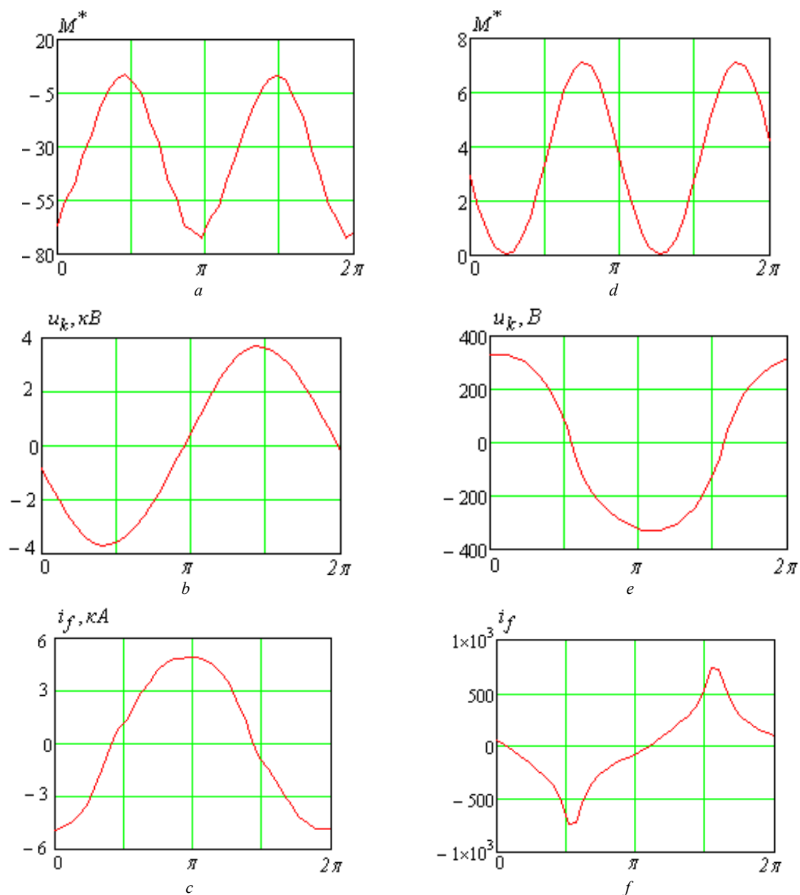
Рис. 2. Періодичні залежності електромагнітного моменту, напруги на конденсаторі та струму збудження при ковзанні s = 1 і двох значеннях ємності конденсатора в обмотці збудження C = 50 \mu\text{Ф} (a-c) та C = 45 \mu\text{Ф} (d-f)
