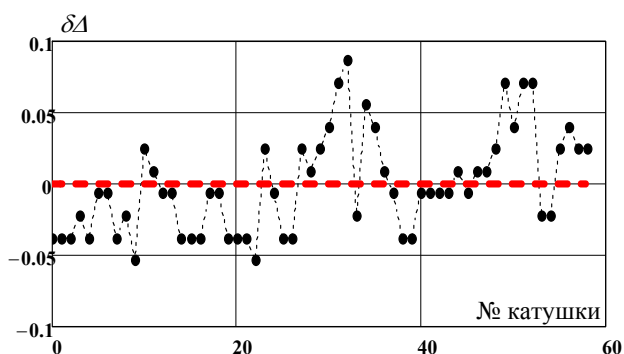
Рис. 3. Относительное изменение диаметральной толщины эмальизоляции \delta A в непрерывном процессе изготовления эмальпровода ПЭИДХ2-200-МЭК диаметром 0,56 мм
