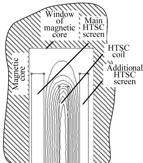
Рис. 3. Розподіл магнітного поля у вікні магнітопроводу обмежувача струму
