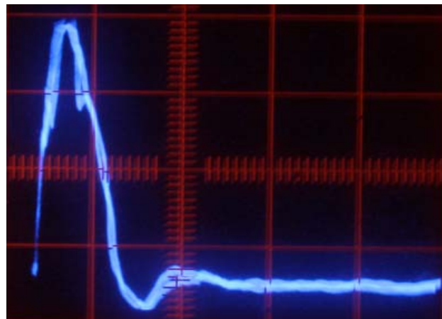
Рис. 5. Осциллограммы (наложено две осциллограммы) импульсов напряжения на нагрузке в виде 10 резисторов ТВО-10 по 560 Ом: цена деления по оси времени 100 нс/дел, по оси процесса 6 кВ/дел
